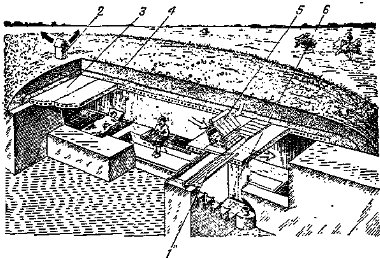
Рис. 8. Противорадиационное укрытие с перекрытием из железобетонных плит:
