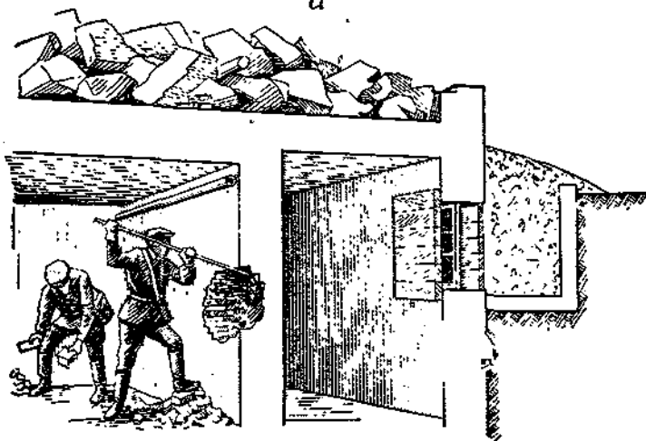
Рис. 23. Выход людей из убежища при завале основного входа.
