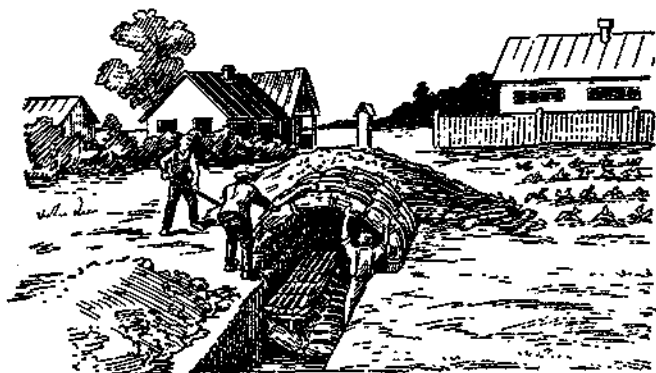
Рис. 9. Устройство противорадиационного укрытия из кольцевых фашин
